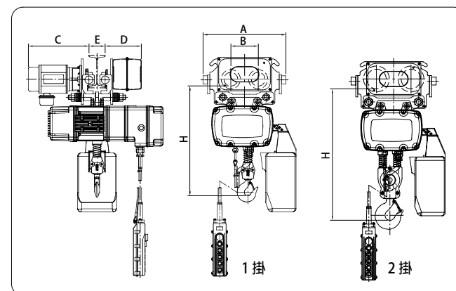
主機配合小車
