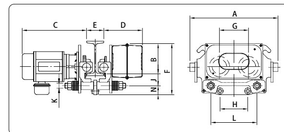
電動小車
